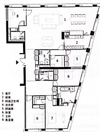
原始平面图
